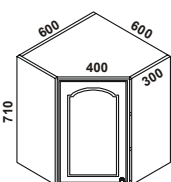
HRS40-B+P40/71+K4 Horní roh dveře šíře 400
