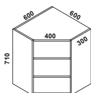
HRS40-B Horní korpus-roh dveře šíře 400
