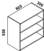
HD60 - korpus nad digestoř snížený
