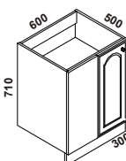
SRP30/P + P30/71 + K2
