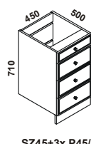
SZ45+3x P45/13+P45/32 +3xM2 + 1xM3
