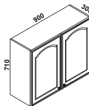
H90 + 2xP45/71 + 2xK1
