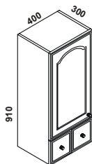
HP 40+P40/71+K1+ 2xP20/20+2xZ20/20 prodloužený zásuvky
