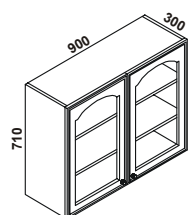
H90 + 2xPP45/71 + 2xK1
