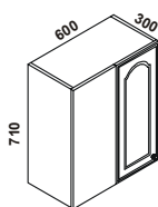
HRP30/P+P30/71+K2 Horní roh-přímý dveře šíře 300
